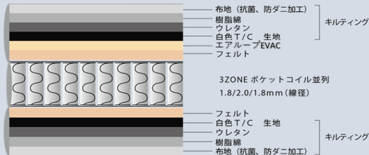
断面図
